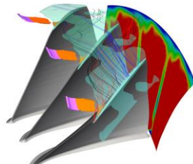
Rotorspaltleckageströmung
